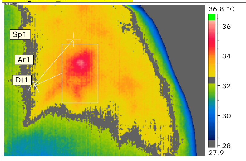
Thermogram: IR_0942.JPG 2/23/2007
